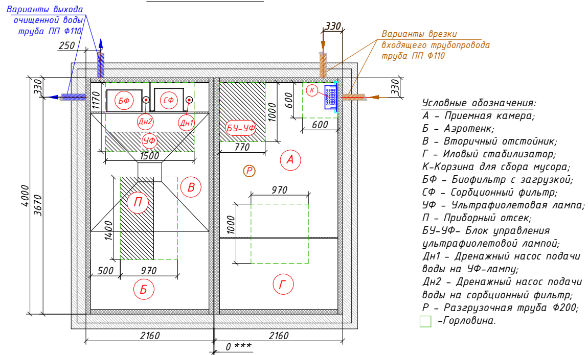
Схема станции
