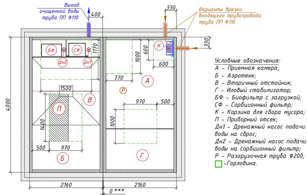
Схема станции
