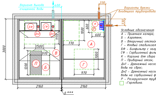
Схема станции
