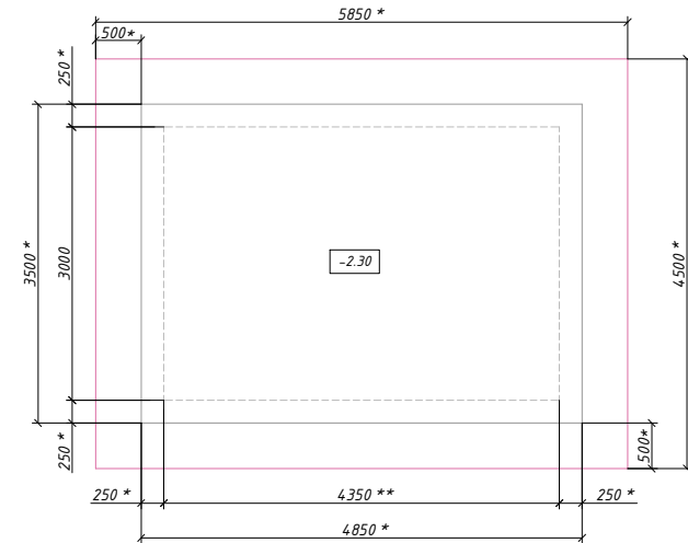
План котлована с плитой
