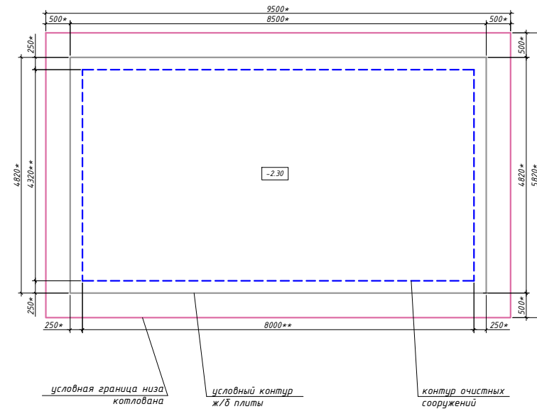
План котлована с плитой
