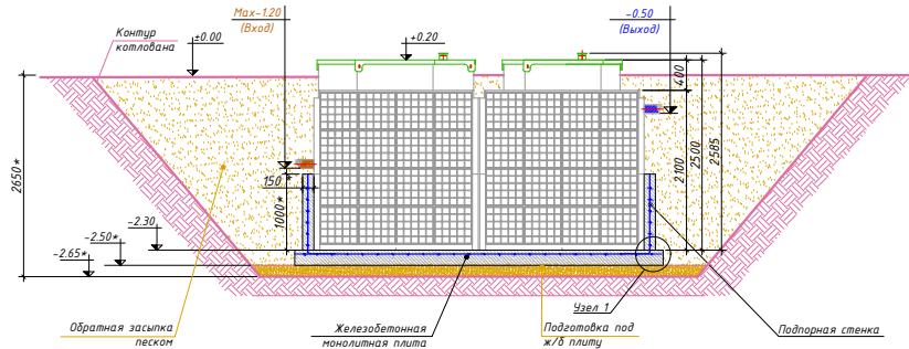
Станция в разрезе котлована
