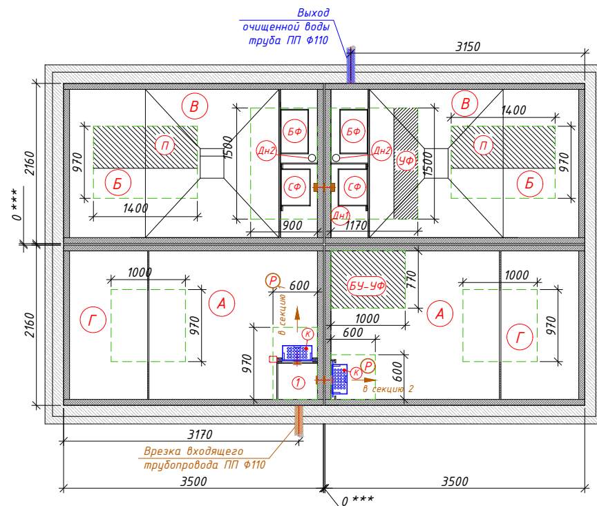
Схема станции
