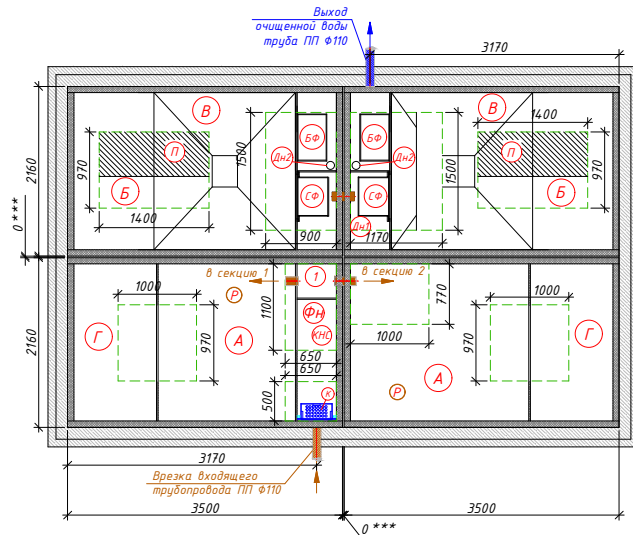
Схема станции
