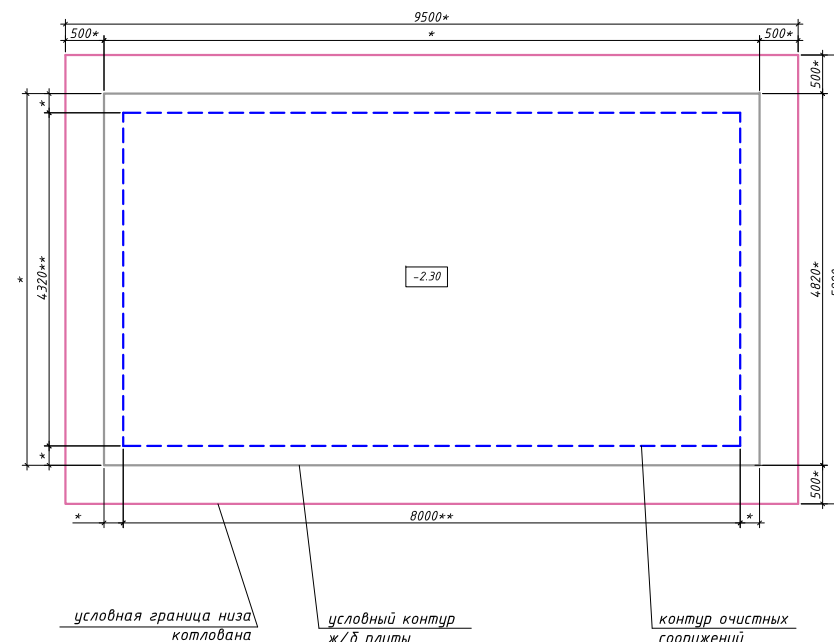
План котлована с плитой
