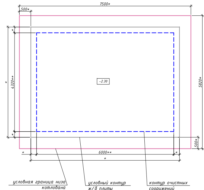
План котлована с плитой
