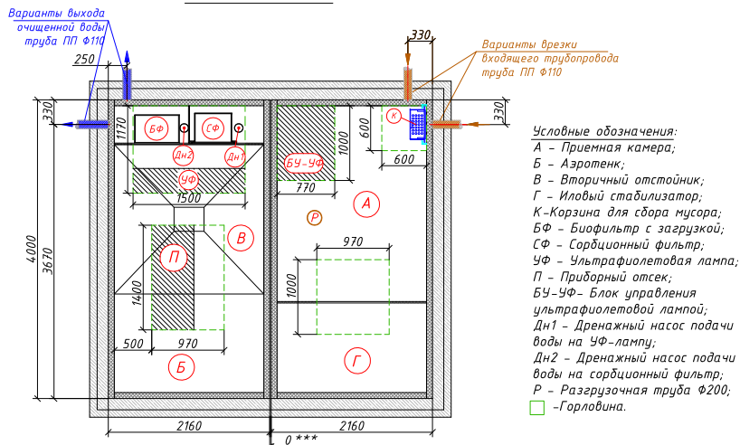
Схема станции
