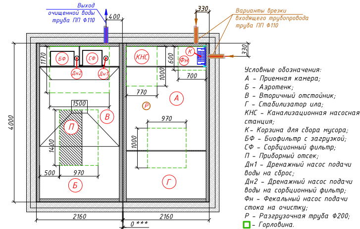
Схема станции
