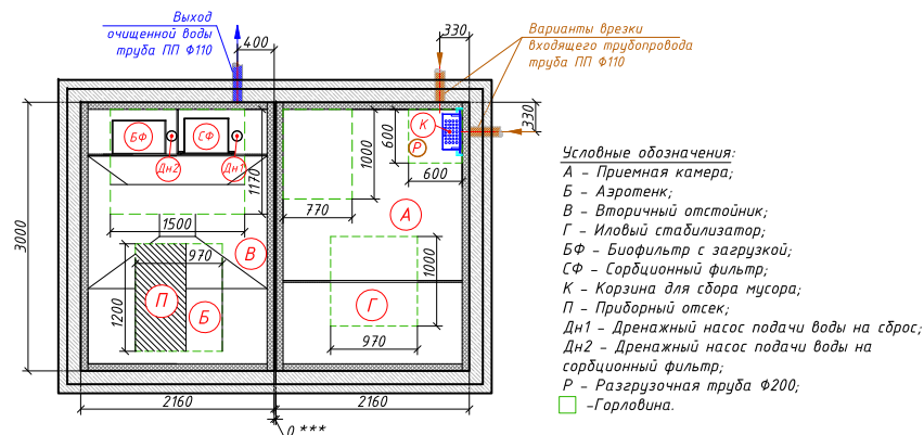
Схема станции
