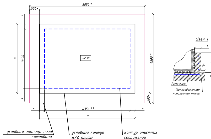
План котлована с плитой
