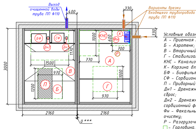
Схема станции
