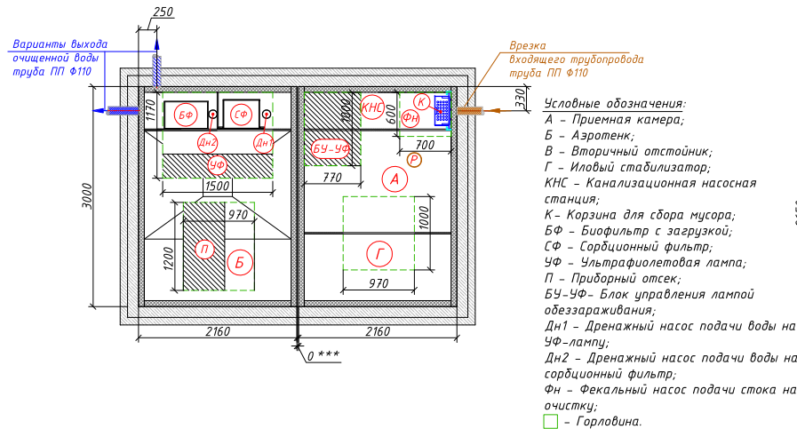
Схема станции
