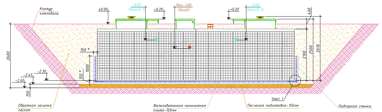
Станция в разрезе котлована
