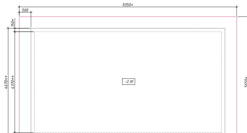
План котлована с плитой
