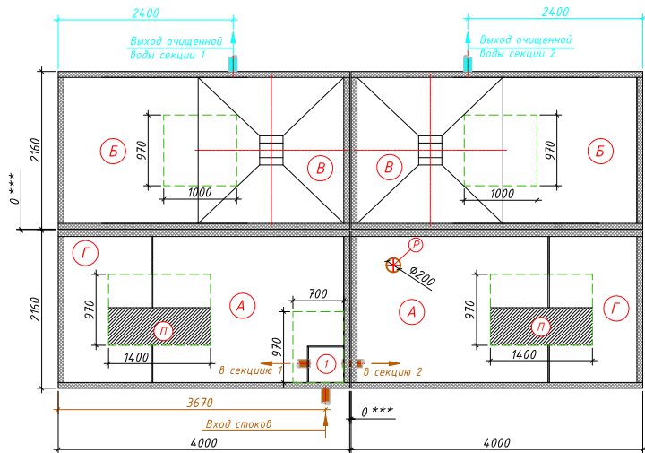
Схема станции
