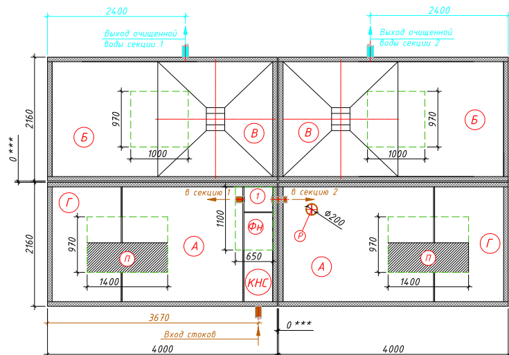
Схема станции
