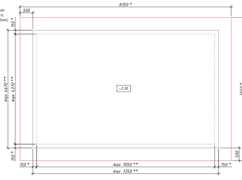
План котлована с плитой
