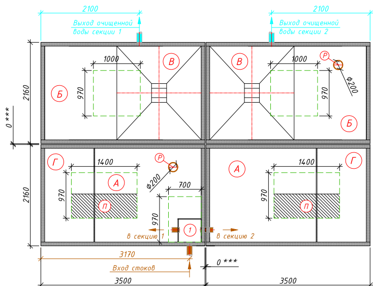
Схема станции
