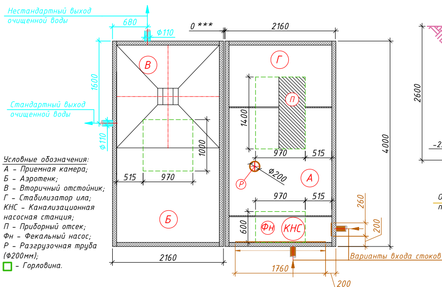
Схема станции
