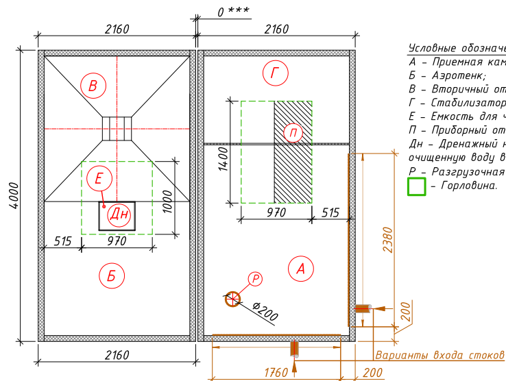
Схема станции
