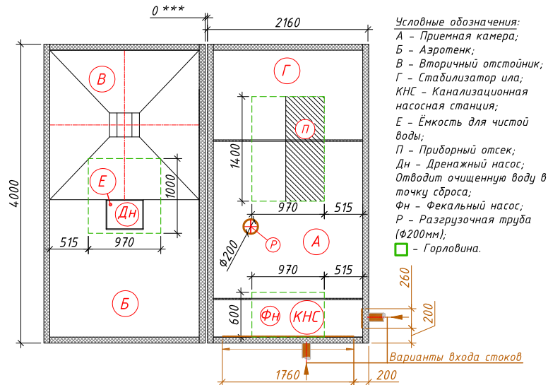
Схема станции
