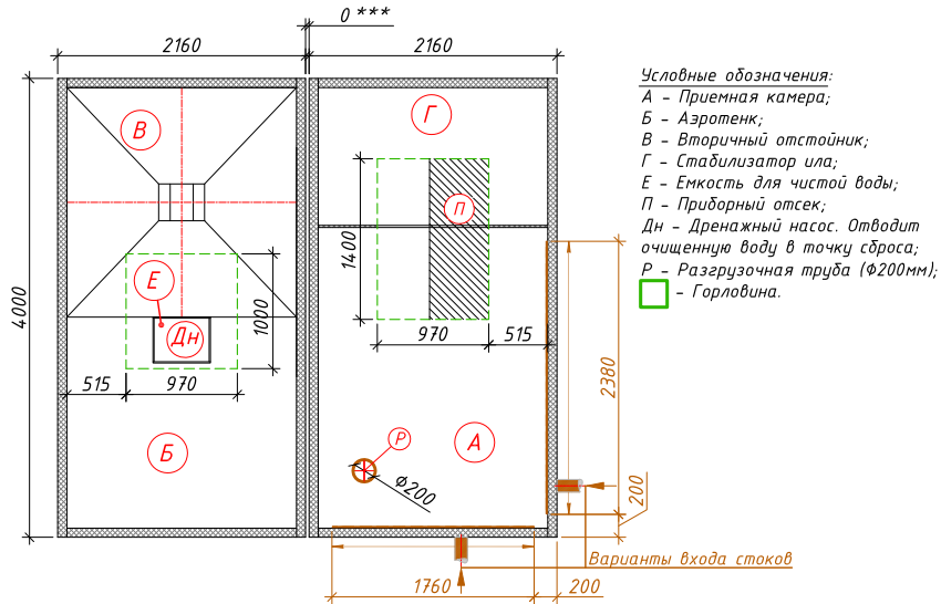
Схема станции
