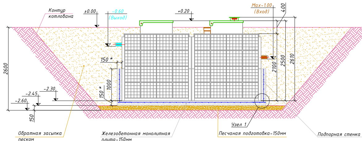
Станция в разрезе котлована
