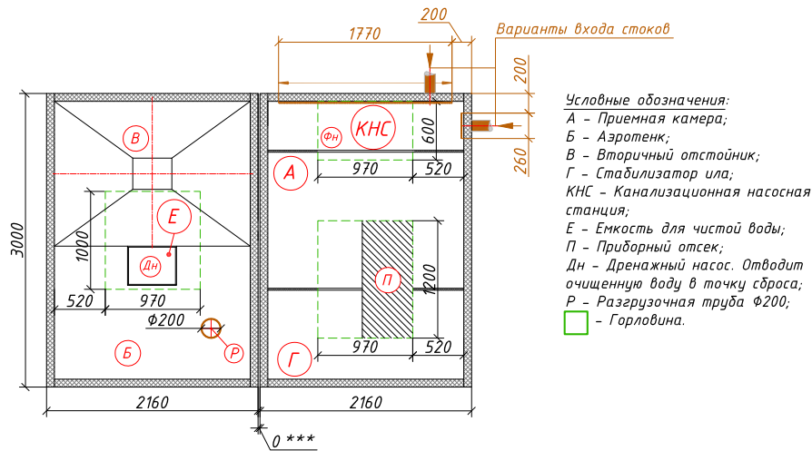
Схема станции
