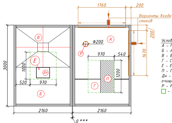
Схема станции
