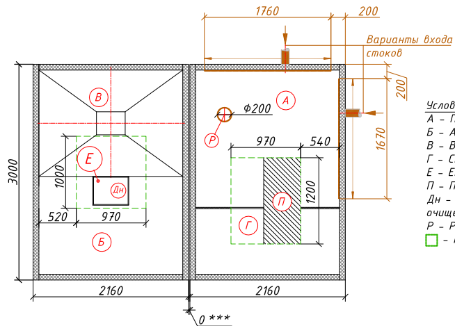
Схема станции
