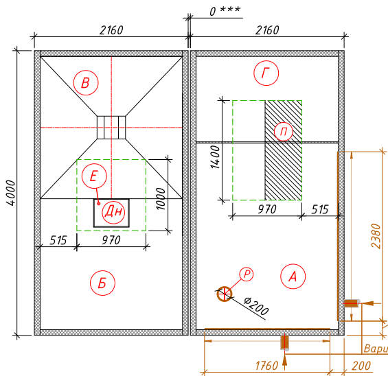
Схема станции
