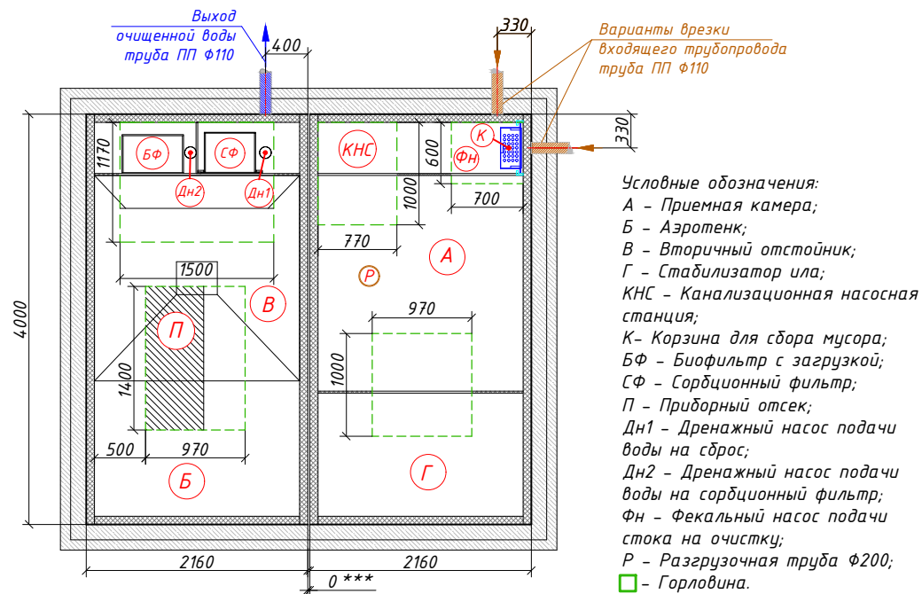
Схема станции
